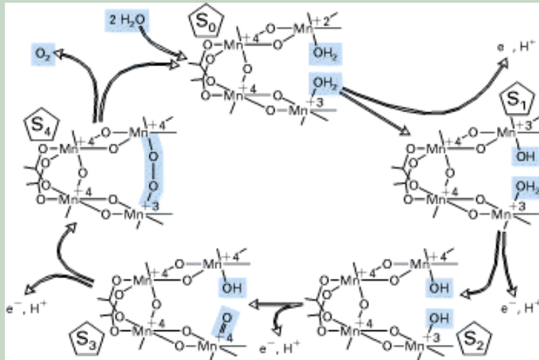
Modelo del ciclo S del complejo productor de oxígeno en el centro de reacción del PSII de un cloroplasto.
