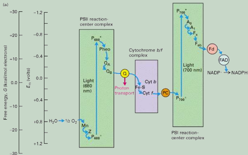
El proceso del flujo electrónico lineal, en donde PSI y PSII están acoplados, genera O_2 , NADPH y un gradiente de protones a través de la membrana tilacoide.
